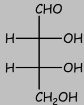
D-Erythrose
