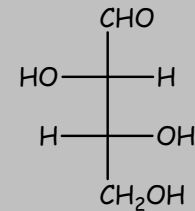
D-Threose
