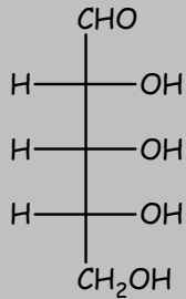
D-Ribose
