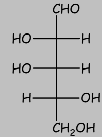
D-Lyxose
